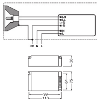
Technische Daten Osram LED Treiber PowerTronic FIT 35/220 240 S
